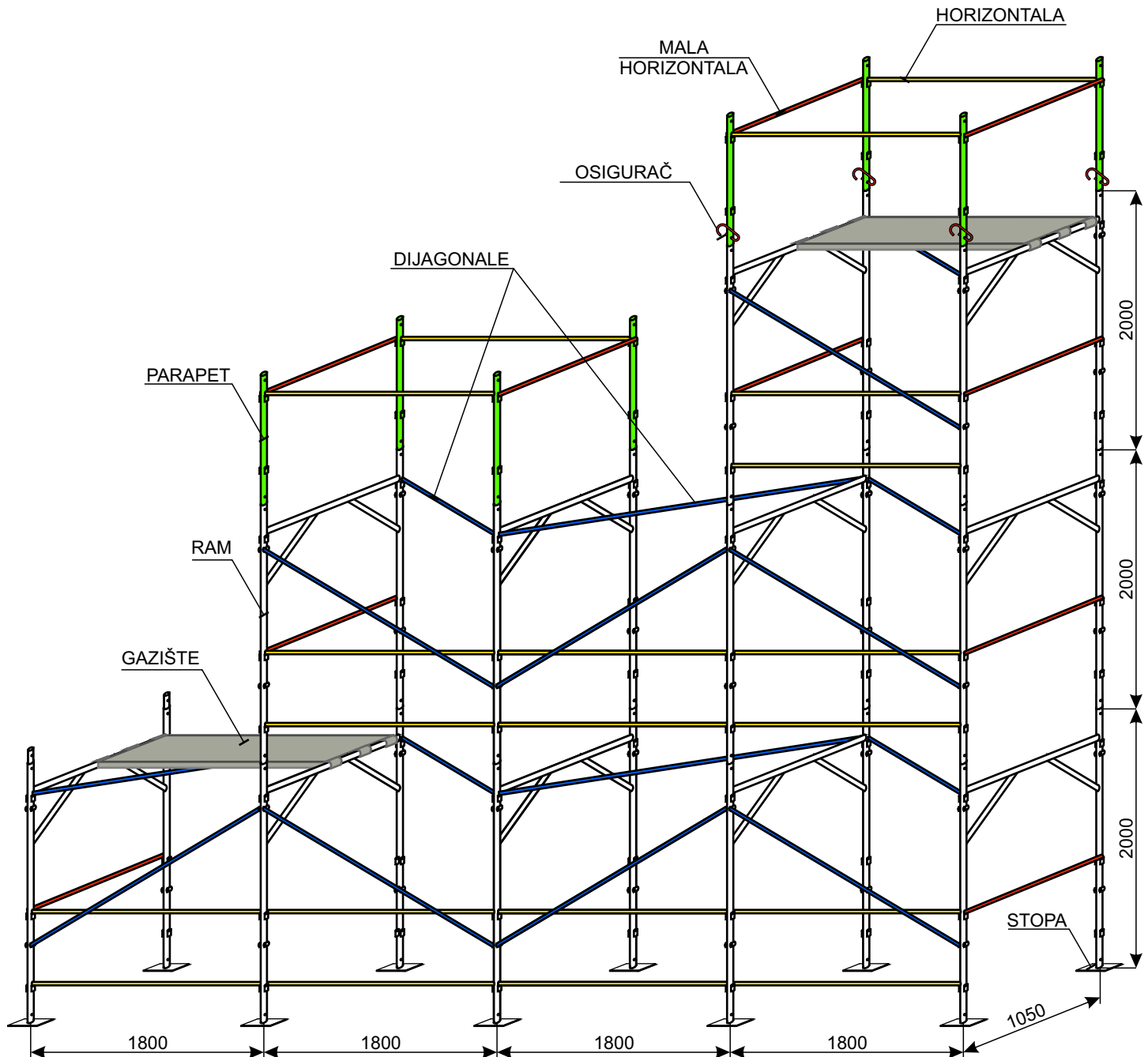
Slika 1. PRIMER MONTAŽE RAMOVSKJE SKELE TIPA "BOCCOLE"
